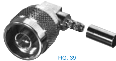
FIG. 39 RT-1009-C1-03
