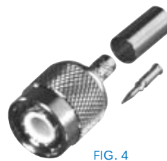
FIG. 4 RFT-1202-2, -2T, -2TC1, -C1, -C2, -C2T
